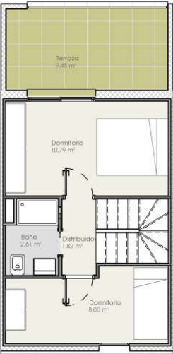
PLANTA PRIMERA
